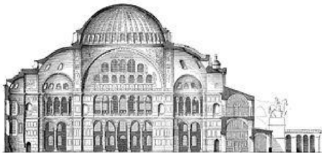
Coupe de Sainte-Sophie
