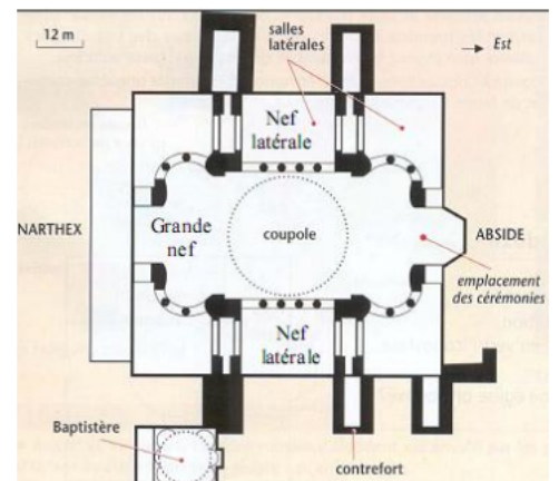
Plan de Sainte-Sophie sous Justinien
